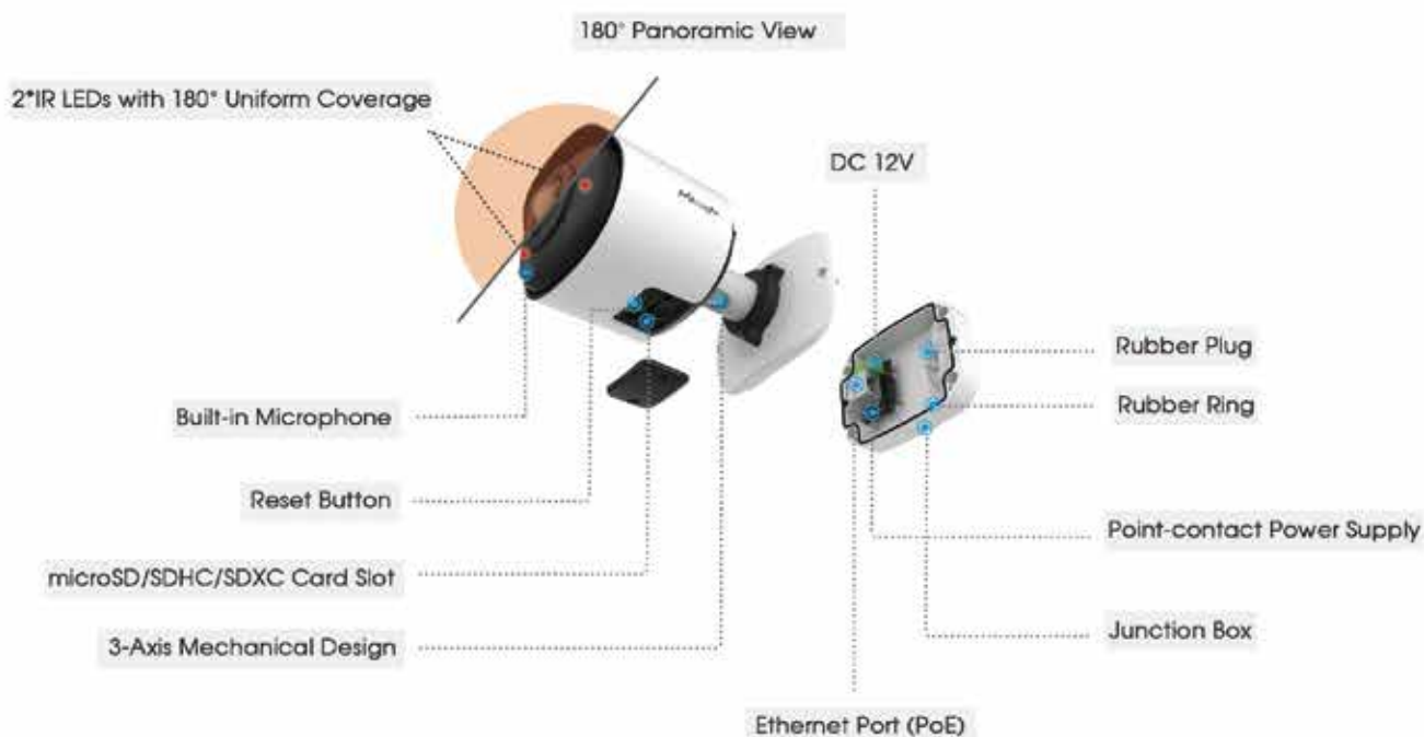
(Mlesight AI 180° Panoramic Mini Bullet Camera)
